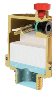
Vanne en position OUVERTE
